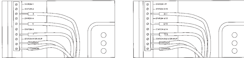
WIRE LAYOUT LEIT 4000 E
